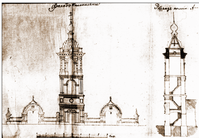
Проект ограды и надстройки колокольни Покровской церкви. 1900 г. Техник архитектуры Н. Жуков.
